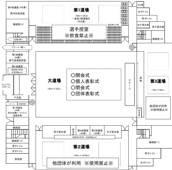
ALSOKぐんま武道館 1階平面図
